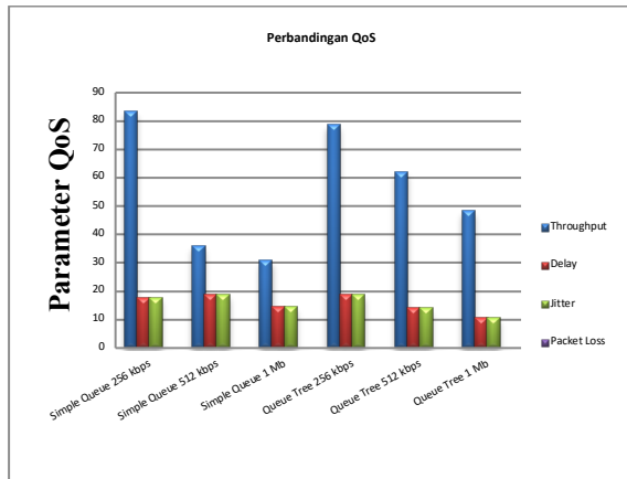
Gambar 12. Grafik Perbandingan Parameter QoS Simple Queue dan Queue Tree
