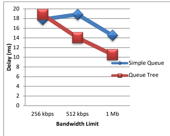
Gambar 9. Grafik Perbandingan Delay
