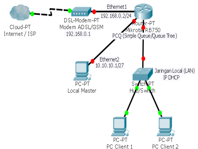
Gambar 2. Desain Jaringan
