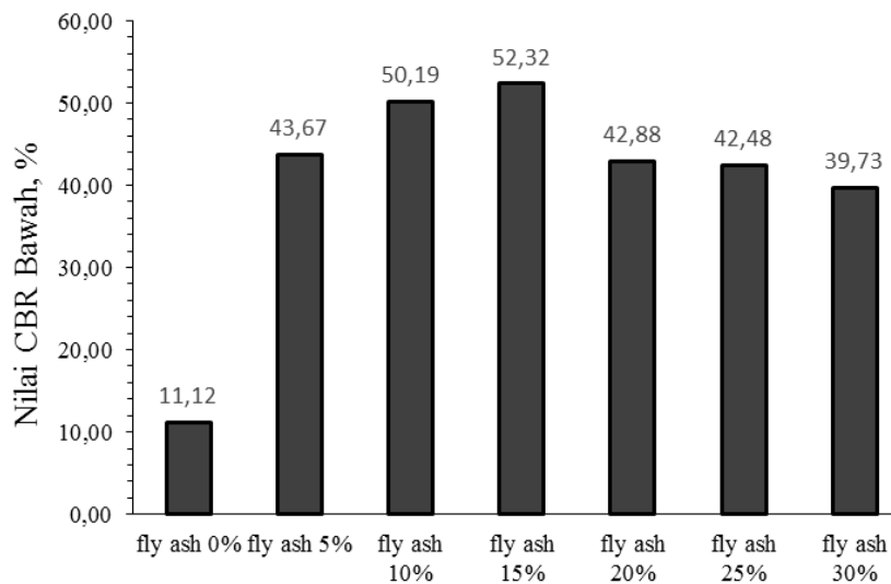
Gambar 7. Korelasi Nilai CBR Bawah Terhadap Penambahan Bahan Additive
